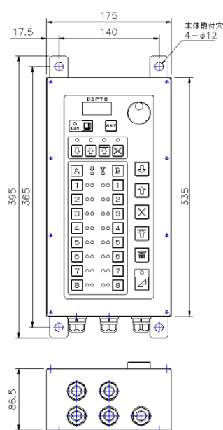
単独操作盤外形図
