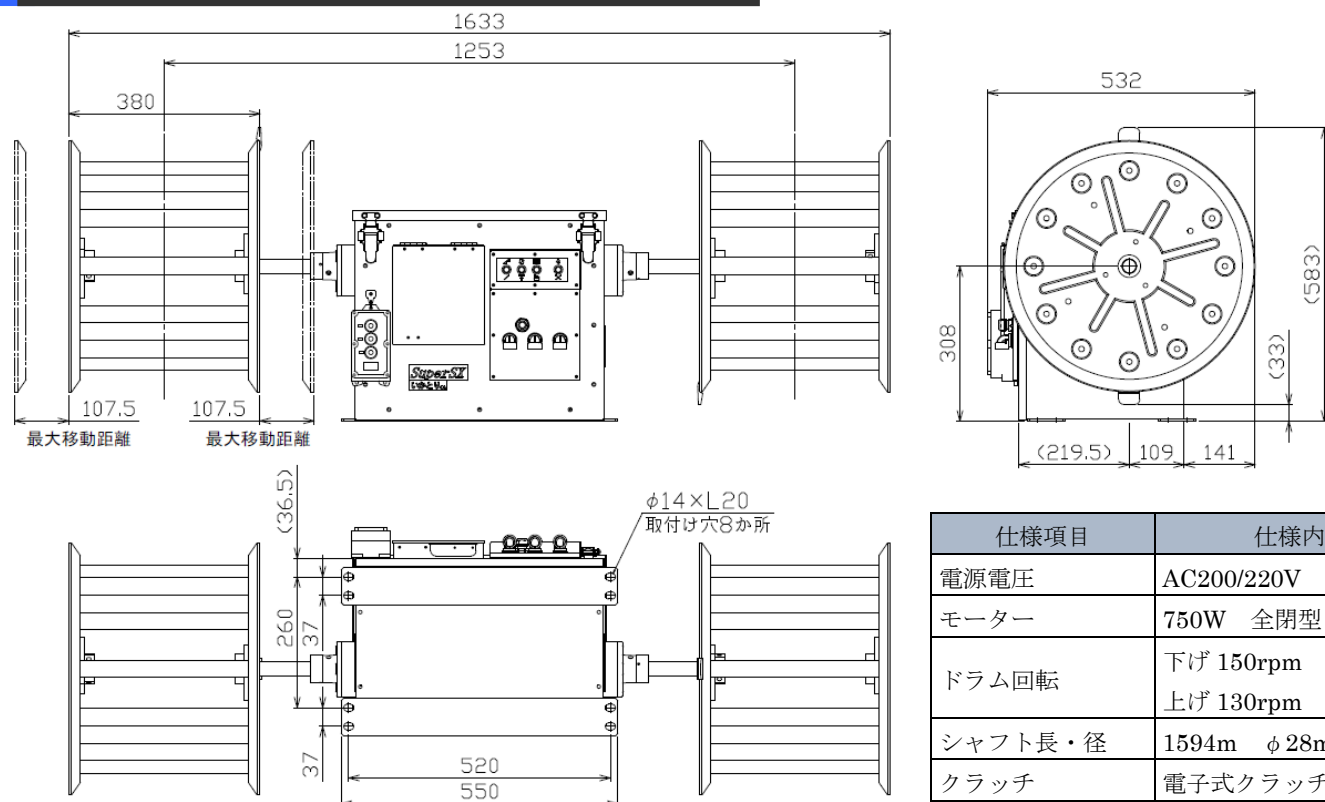
釣り機外形図
