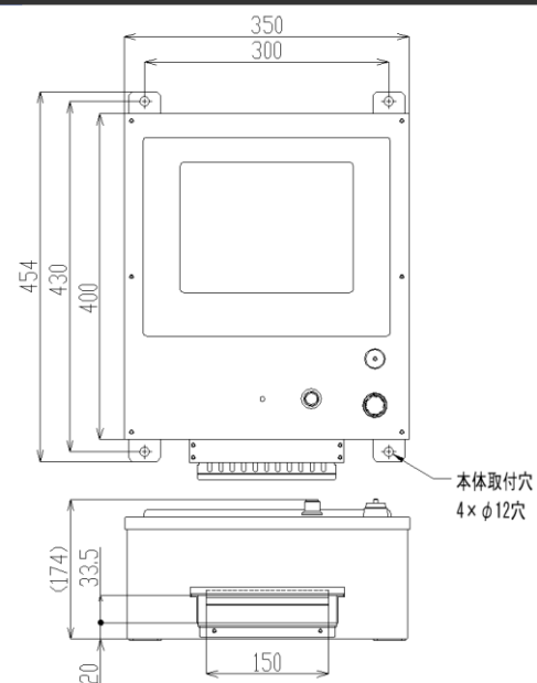
集中制御盤外形図
