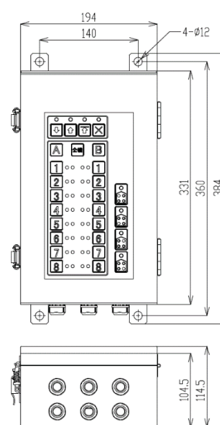
警報操作盤外形図
